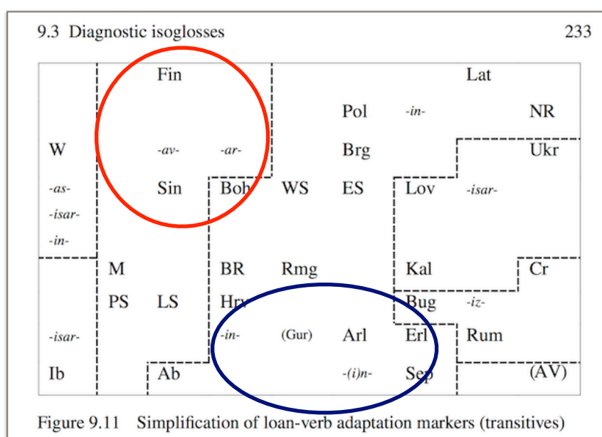
Schematiskt uppställning av markör för låneord i olika romanivarieteter.
